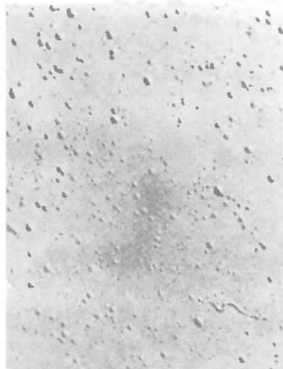
Figura A.7 – Grau de empolamento d 3/t 4
