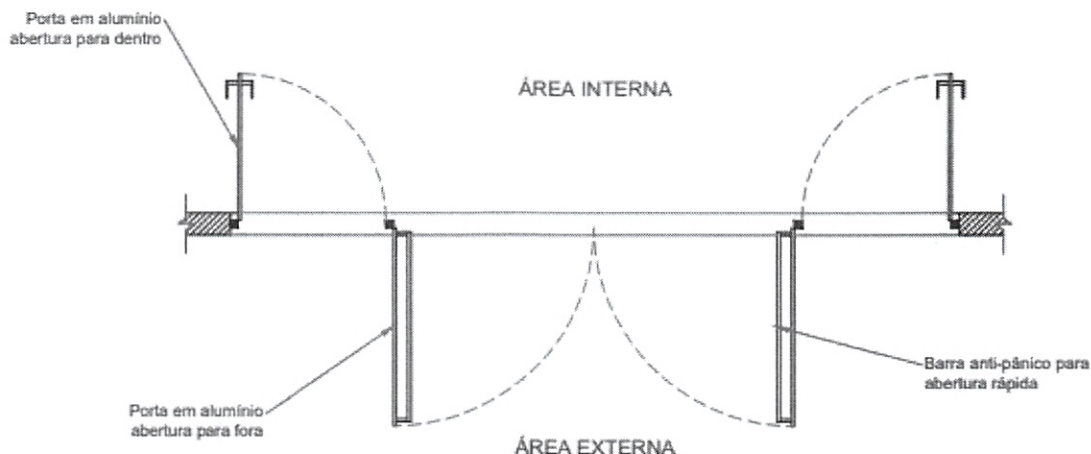
DETALHAMENTO EM PLANTA ESCALA: 1/50
