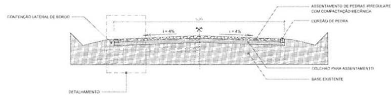
10 SEÇÃO TRANSVERSAL Escala 1:50
