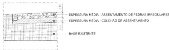
6 DETALHAMENTO PAVIMENTO Escala 1:25
