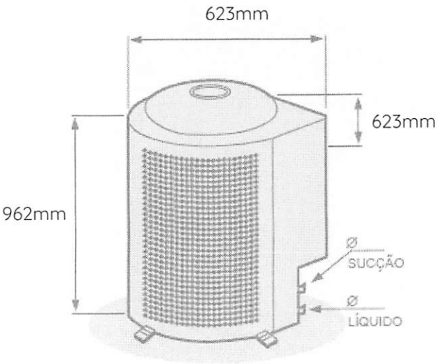
UNIDADE EXTERNA (CONDENSADORA)
