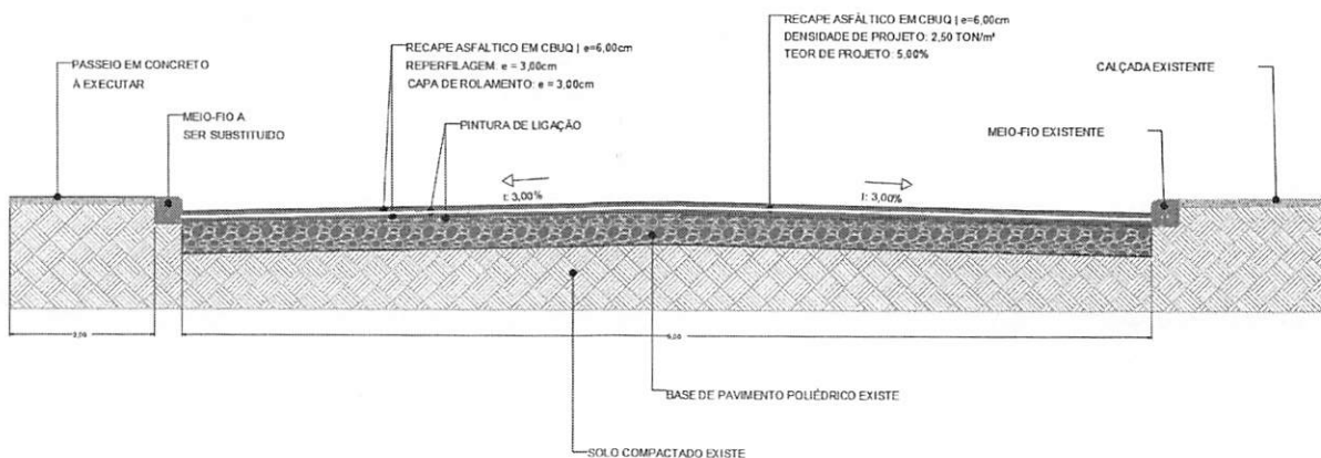
3 SEÇÃO TRANSVERSAL (B-B) SEM ESCALA
