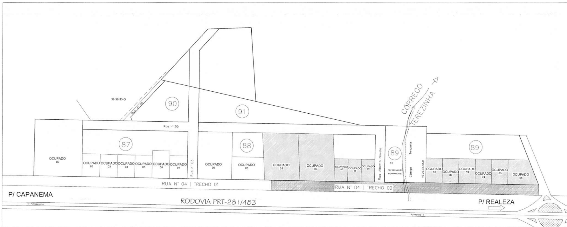
1 LOCALIZAÇÃO DOS LOTES LINDEIROS SEM ESCALA
