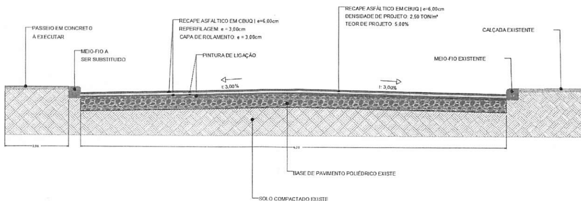
3 SEÇÃO TRANSVERSAL (B-B) SEM ESCALA
