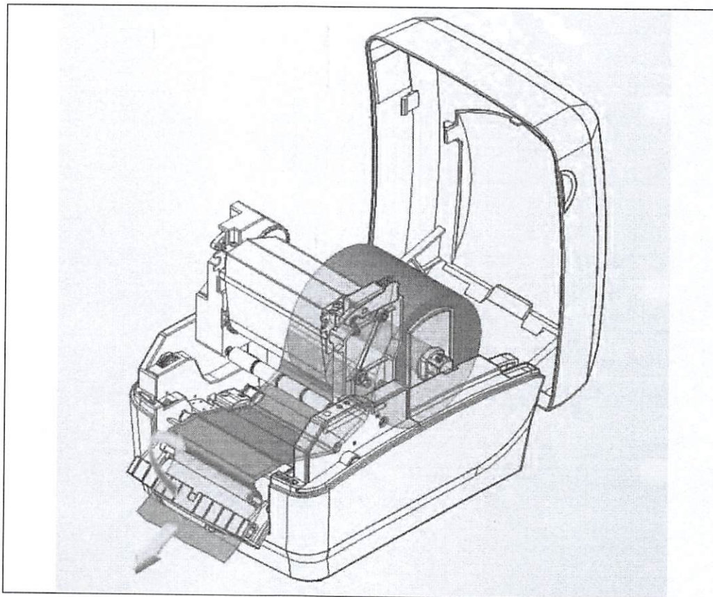
Fig. 11 – Passando o liner pelo mecanismo de Peel Off
