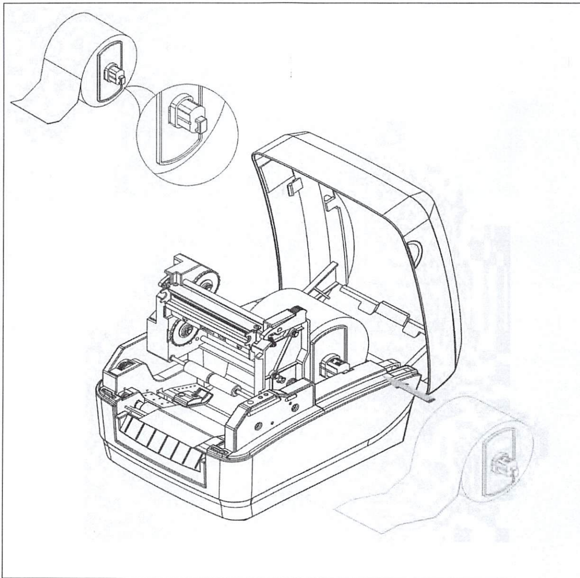
Fig. 7 – Instalando o rolo de papel
