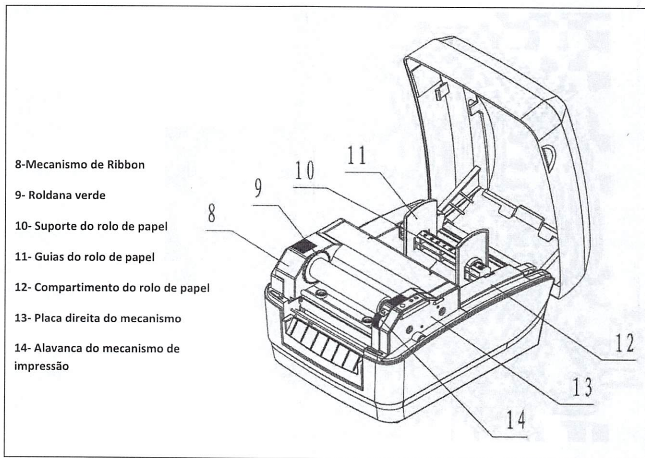
Fig.3 – Interior da L42
