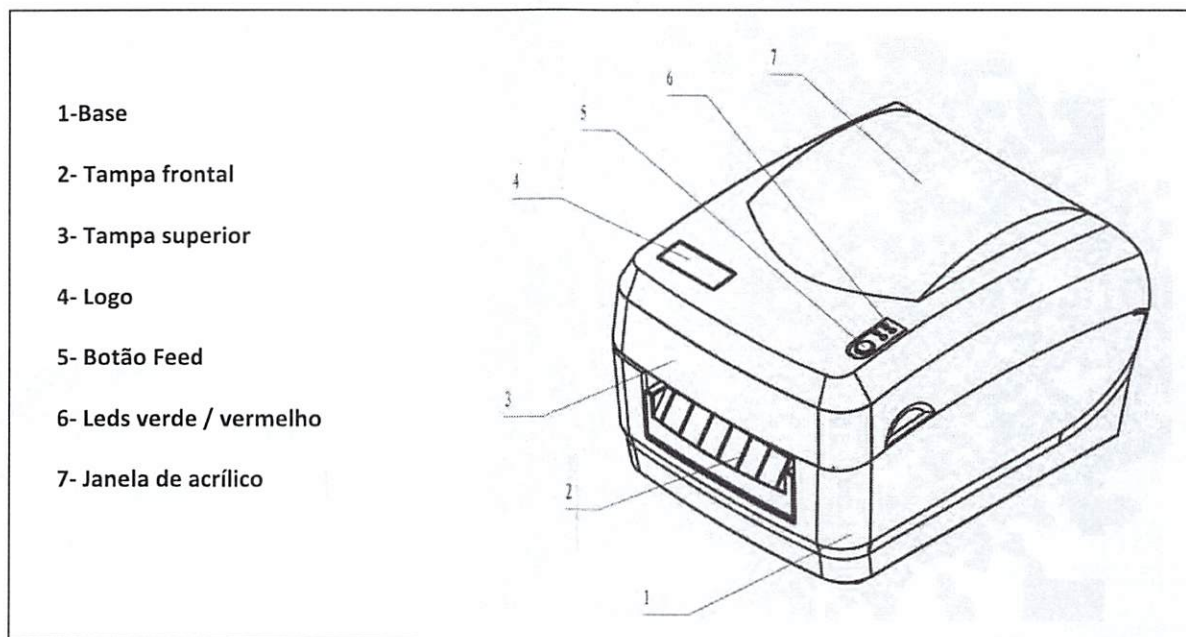
Fig. 2 – Exterior da L42
