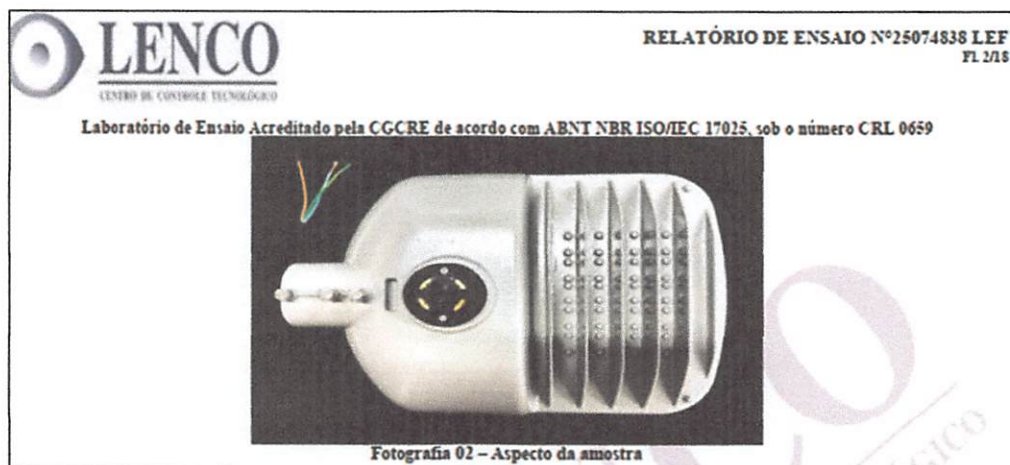
Figura 6 - Luminária de 200W LD 8P-200-4000-170SV, apresentada para validar os ensaios de segurança sob o documento REEME - Luminária Pública LD 8P-200-4000-170-SV - 25074838 LEF.pdf.
