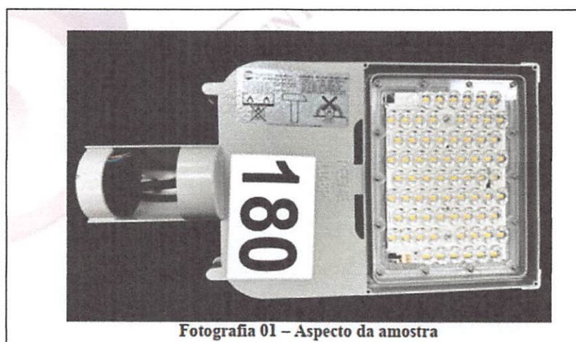
Figura 7 - Luminária de 180W LD 8P-180-4000-170SV sob o REEME - Luminária Pública LD 8P-180-4000-170-SV - 25064728
